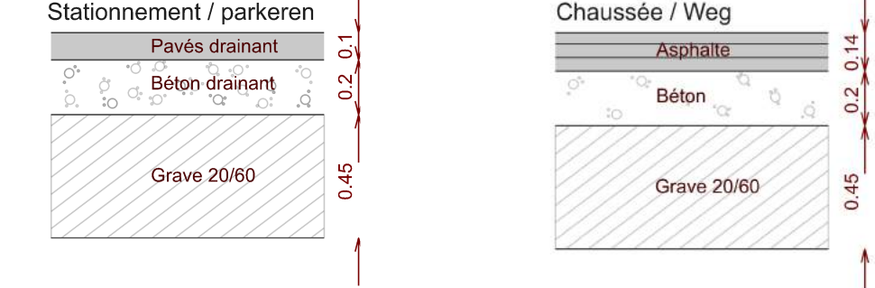
Coupes / Secties
