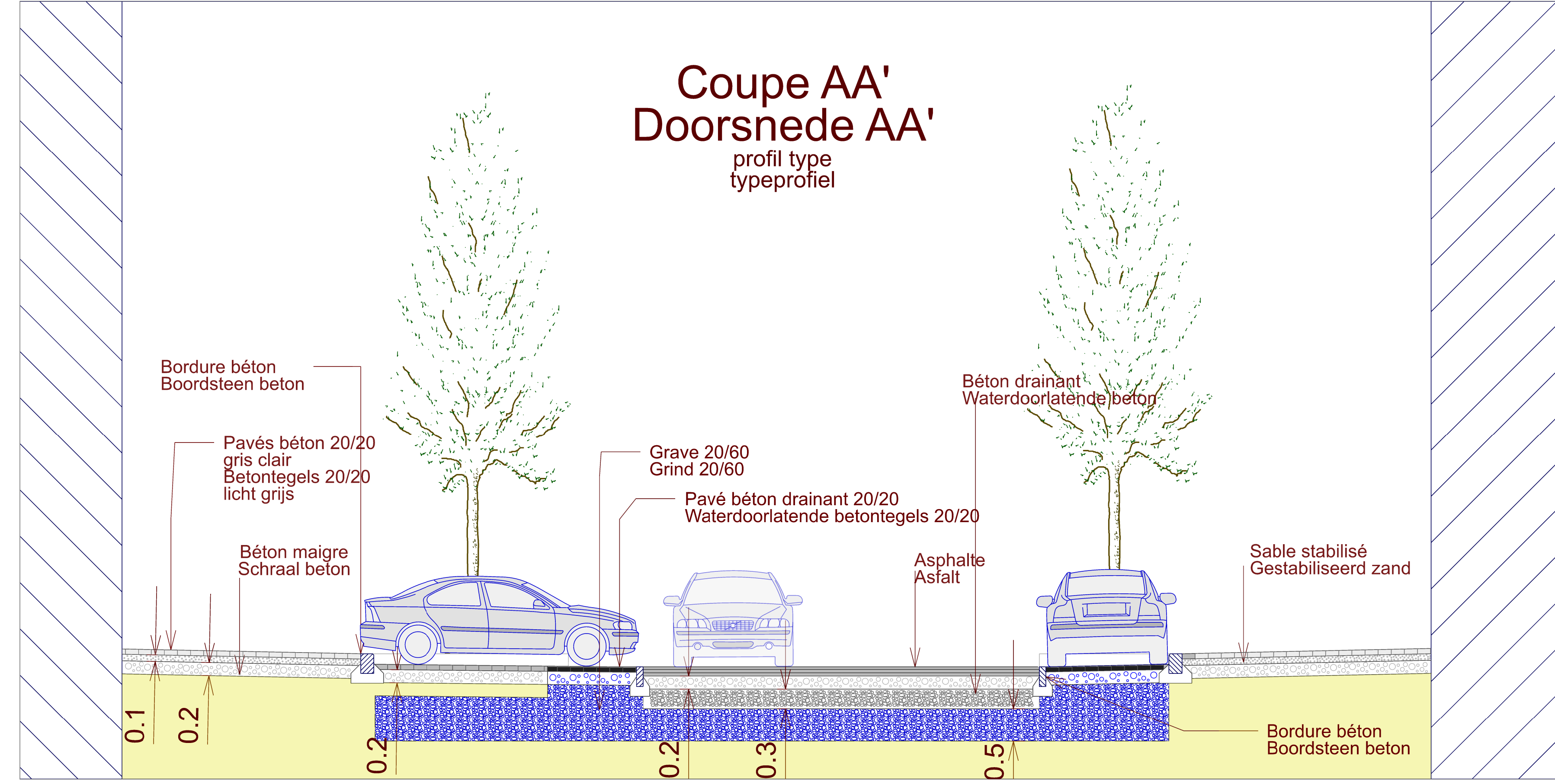
Principe d'infiltration - Echelle 1/50 Infiltratieprincipe - Schaal 1/50
